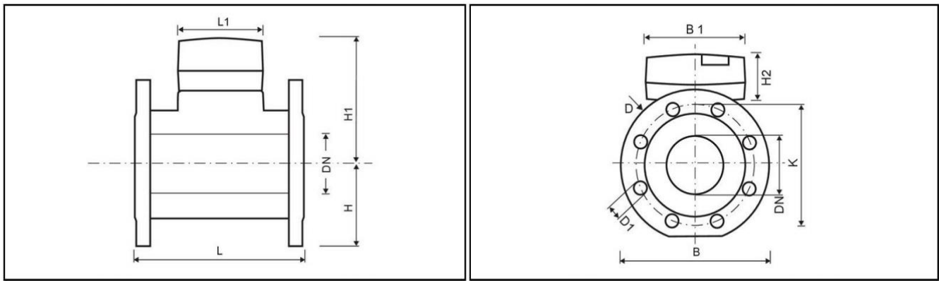
Малюнок 1. Габаритні розміри
