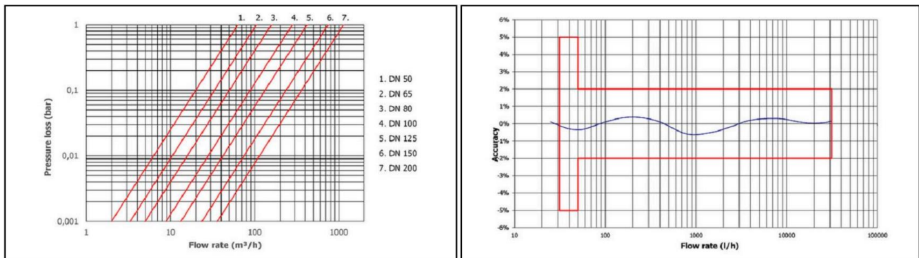
Малюнок 4. Характеристика втрати тиску
