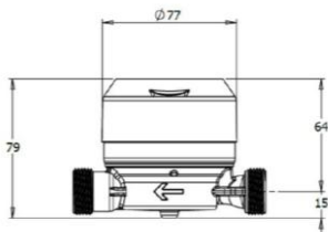
Мал. 1 Лічильник води Aries
